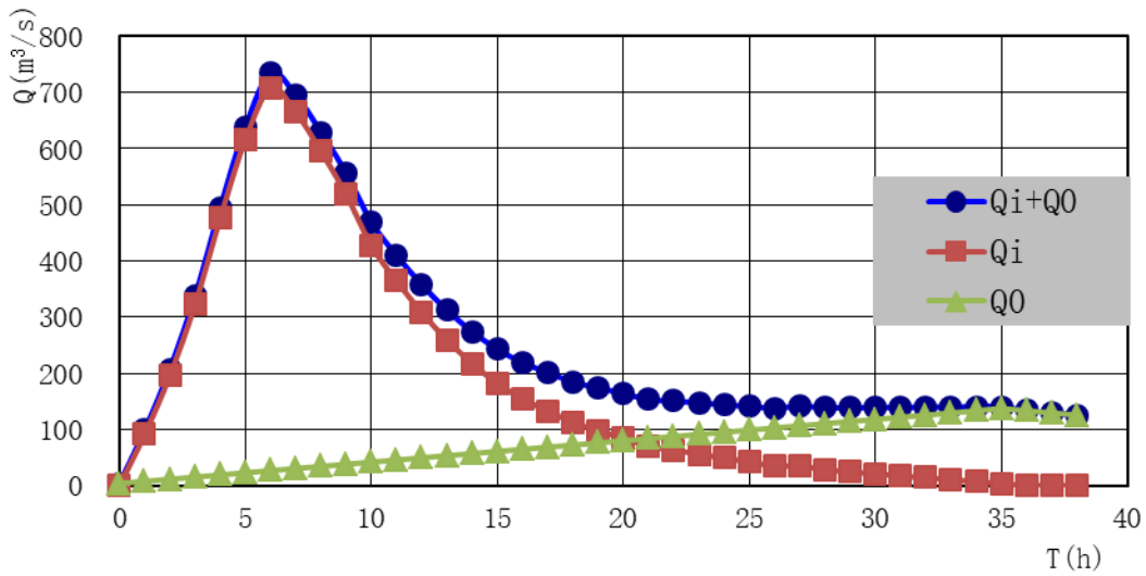
山漳溪十年一遇洪水过程线
