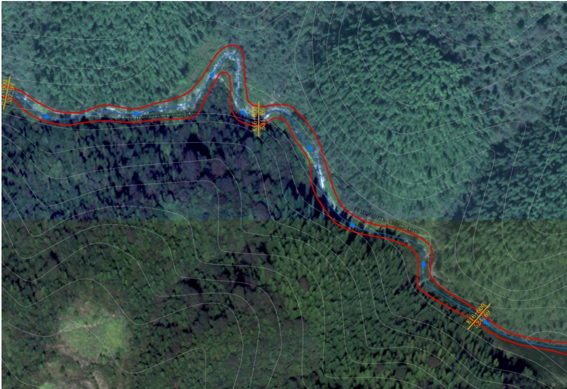
十年一遇设计洪水位线结合自然岸线划定
