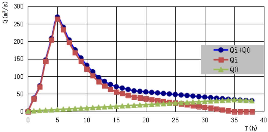
奎溪十年一遇洪水过程线
