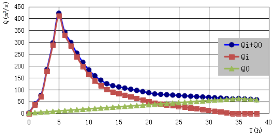
龙溪十年一遇洪水过程线
